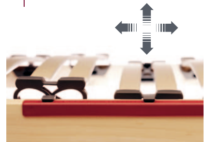
Horizontale und vertikale Einstellungen der Leisten im Schulter- und Beckenbereich für individuelle Anpassung
